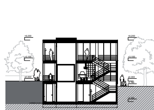
rez BB 1:200
