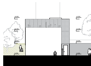
pohľad severný 1:200
