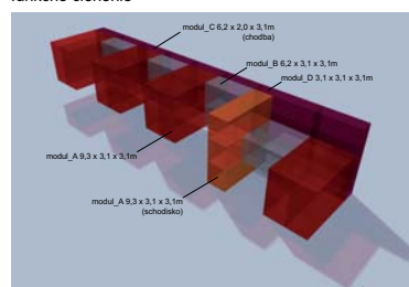
schéma modulov
