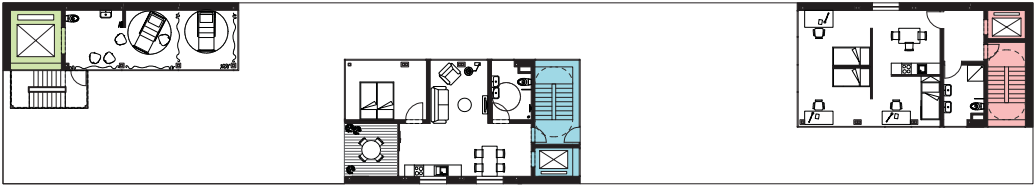
Obytná paluba A (3NP) 1:200
