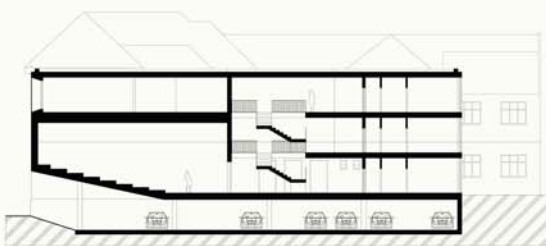
ŘEZ BB
