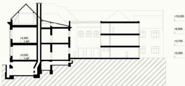
ŘEZ AA
