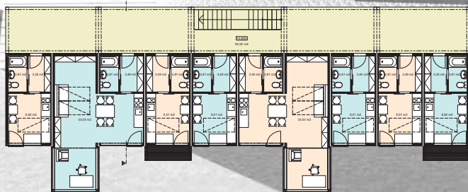
PŮDORYS 3.NP 1:100
