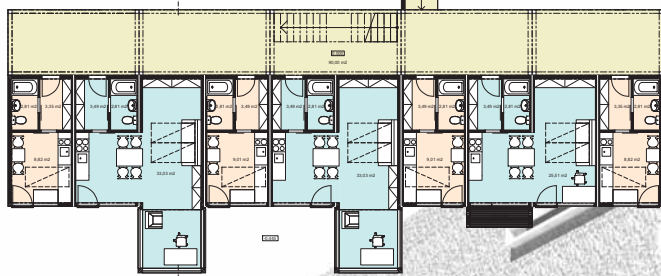
PŮDORYS 1.NP 1:100
