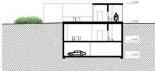
ŘEZOPOHLED JIH 1:250
