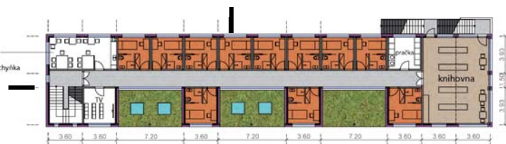
2NP 1:200
