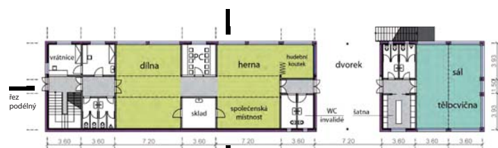
1NP 1:200
