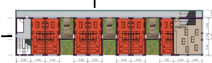
3NP 1:200
