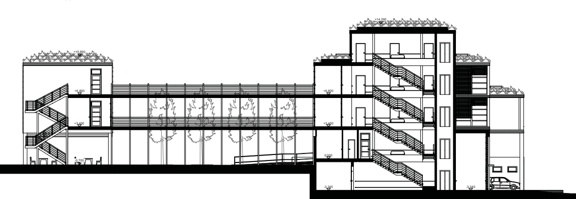
ŘEZ B-B' 1:200
