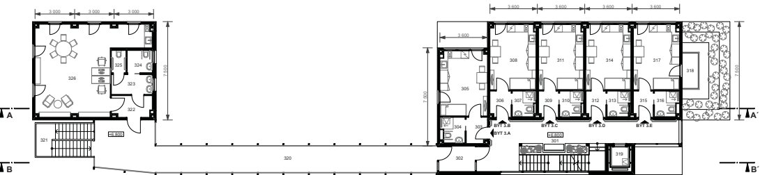
3.NP 1:200
