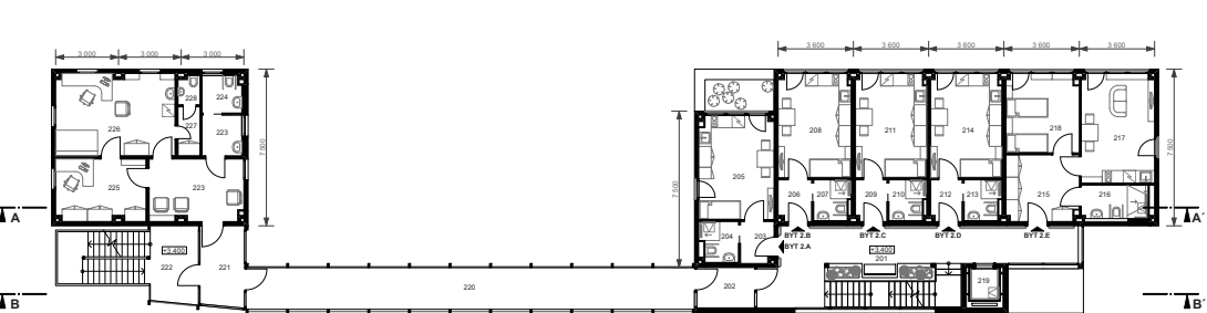
2.NP 1:200
