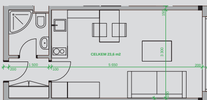
VARIANTNÍ ŘEŠENÍ DISPOZICE BYTŮ, 1 + KK, M 1:50
