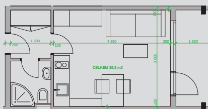
VARIANTNÍ ŘEŠENÍ DISPOZICE BYTŮ, 1 + KK, M 1:50
