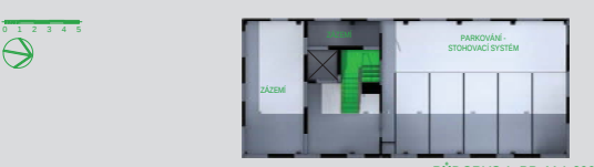
PŮDORYS 1. PP, M 1:200
