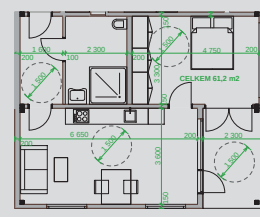
VARIANTNÍ ŘEŠENÍ DISPOZICE BYTŮ, 2 + KK PRO HENDIKEOVANÉ, M 1:100
