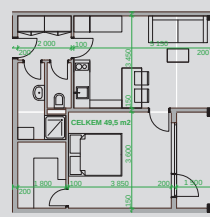
VARIANTNÍ ŘEŠENÍ DISPOZICE BYTŮ, 2 + KK, M 1:100
