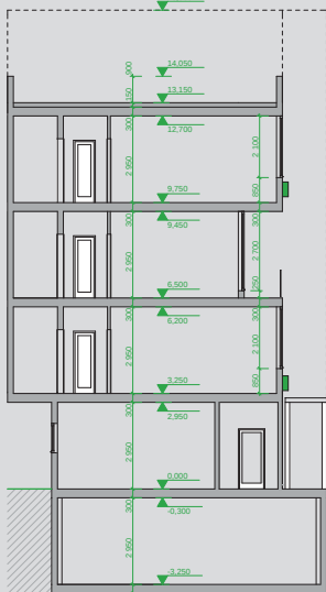
PŘÍČNÝ ŘEZ, M 1:100
