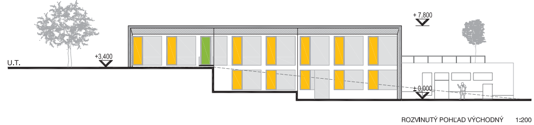
ROZVINUTÝ POHĽAD VÝCHODNÝ 1:200
