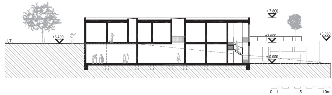
POZDĹŽNY REZ C-C' 1:200
