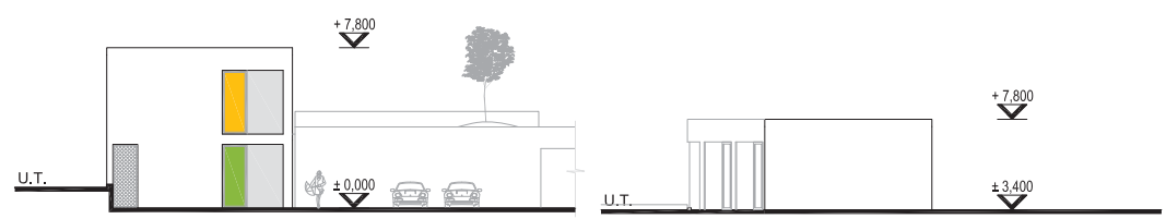
POHĽAD SEVERNÝ 1:200
