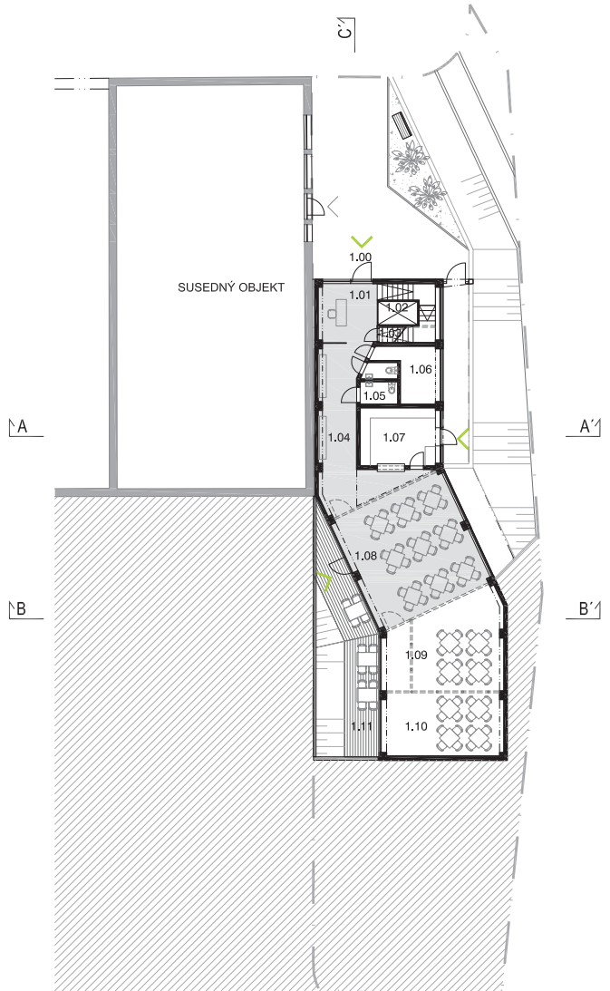
0 1 5 10m PÔDORYS 1. N.P. 1:200
