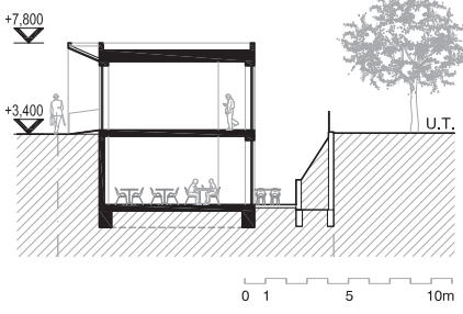
POZDĹŽNY REZ B-B' 1:200
