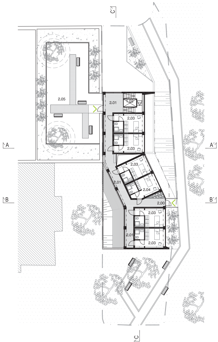
0 1 5 10m PÔDORYS 2. N.P. 1:200
