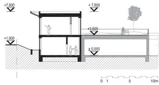
POZDĹŽNY REZ A-A' 1:200
