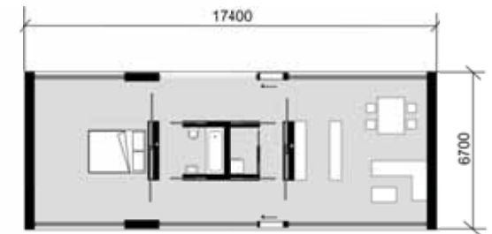
PŮDORYS BUŇKY 1:100
