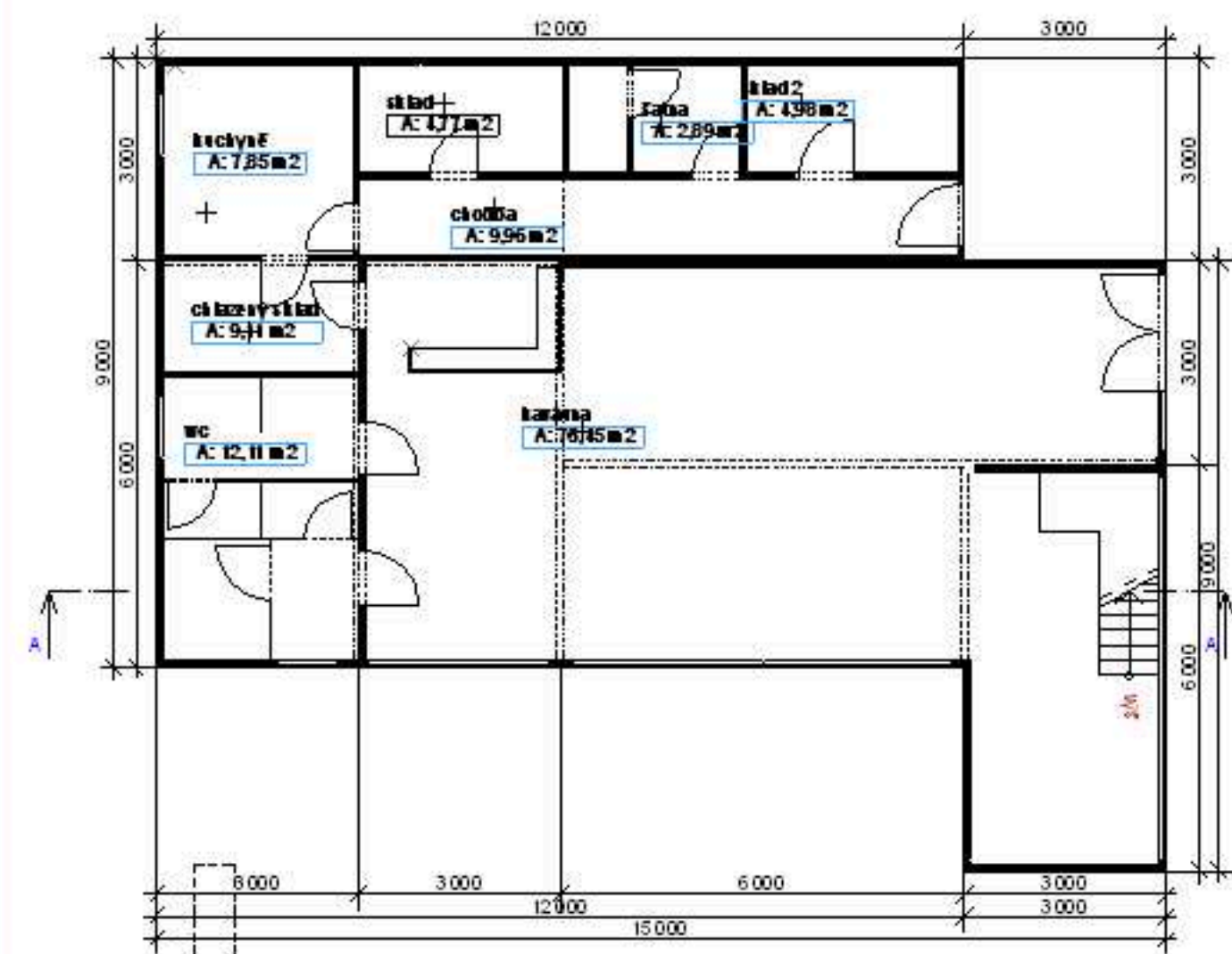
půdorys 1:100, rozdělení na moduly přízemí
